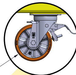
Ø160 x 52 mm avec bandage polyuréthane
